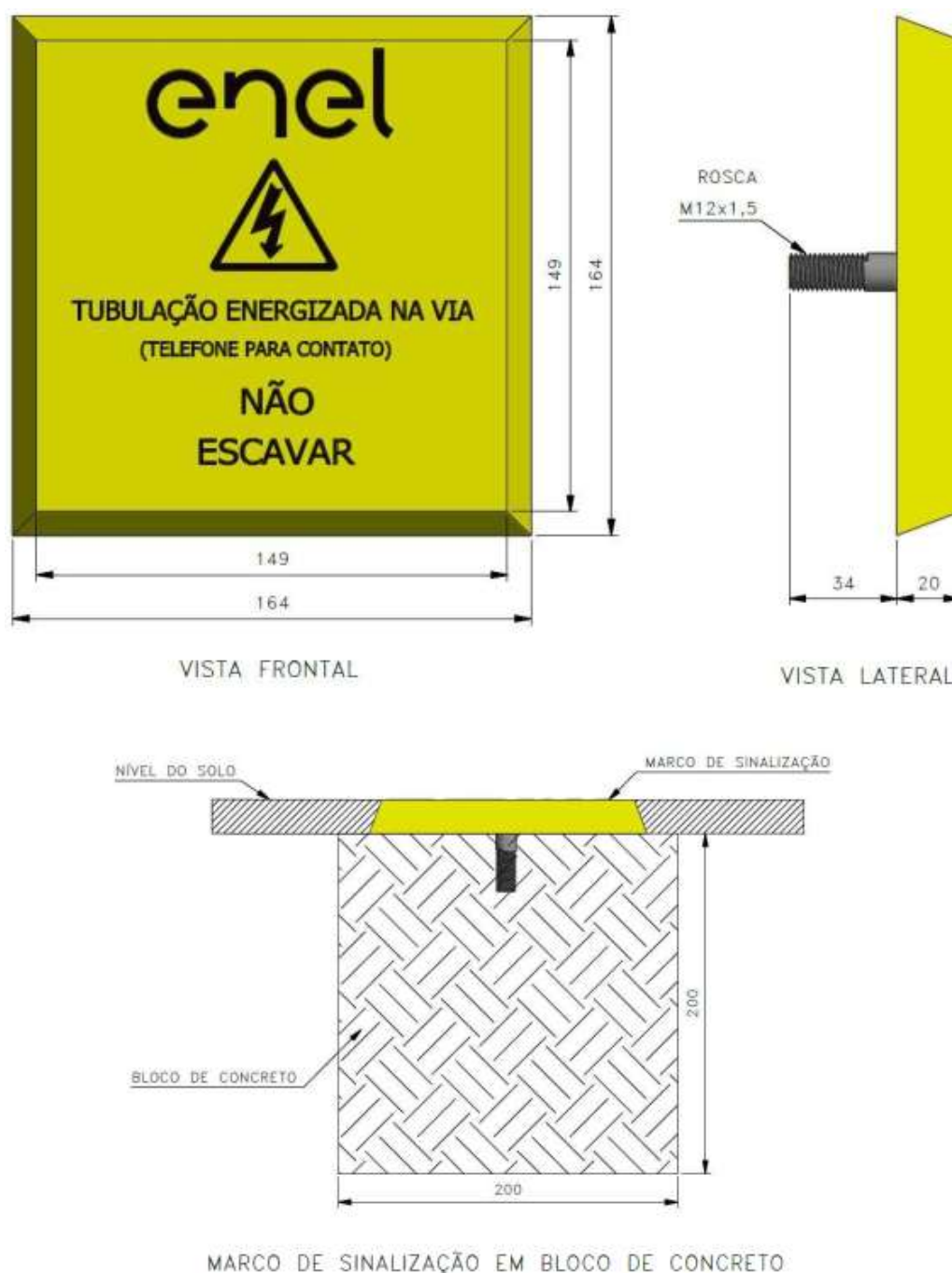
Figura 1 - Marco de Sinalização Horizontal - TIPO 1
